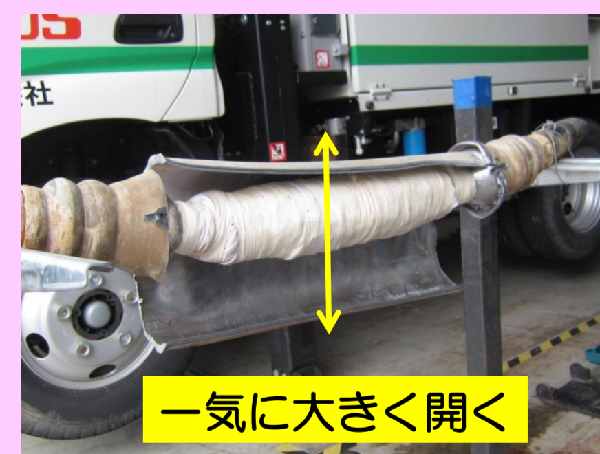
③主鉛管の除去
