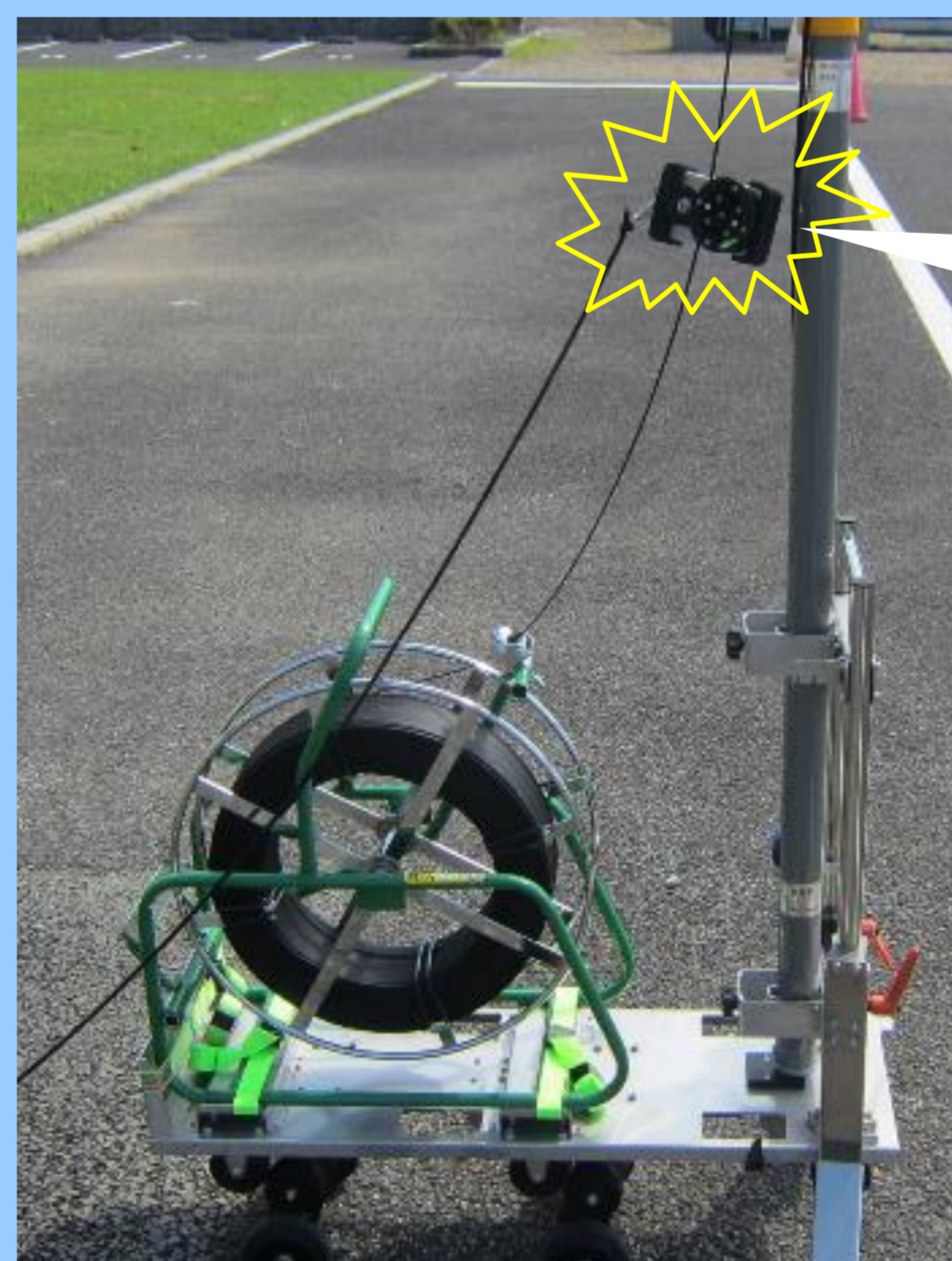
③引込線引き寄せツールを光ドロップに取り付け
